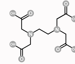
Disodium EDTA
